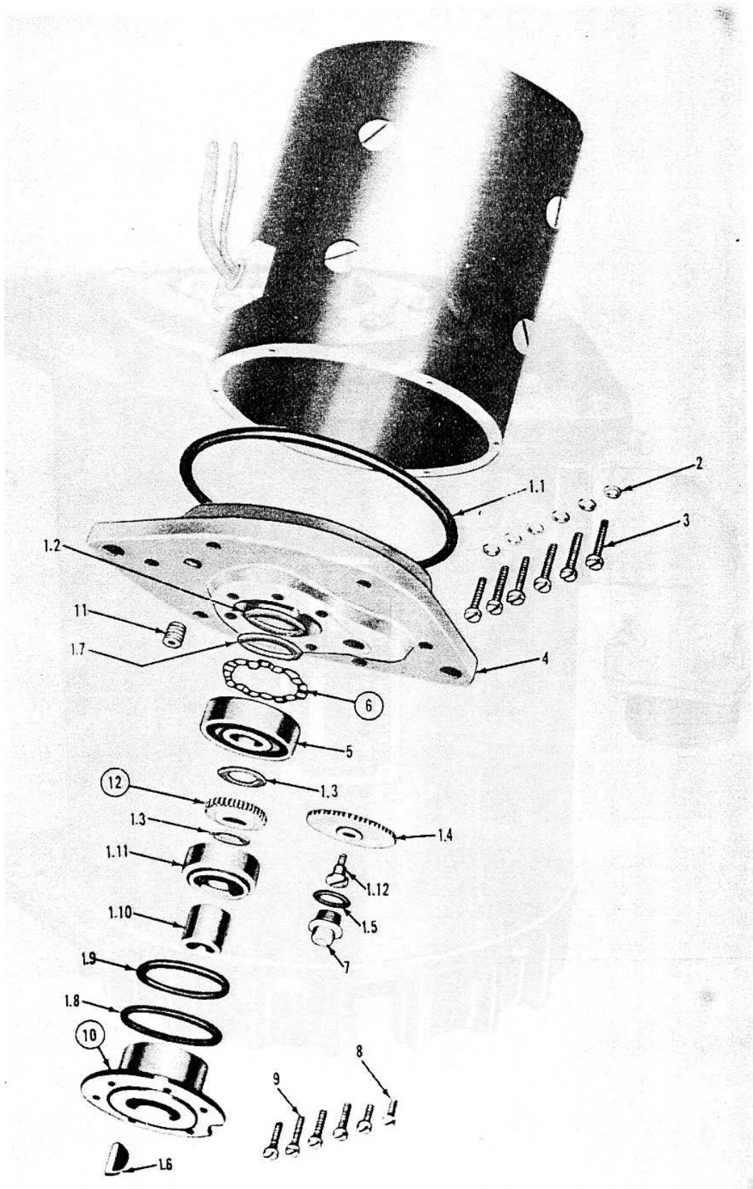
Afb. 2 - GENERATOR, VERBRANDINGSMOTOR (aandrijfzijde)
